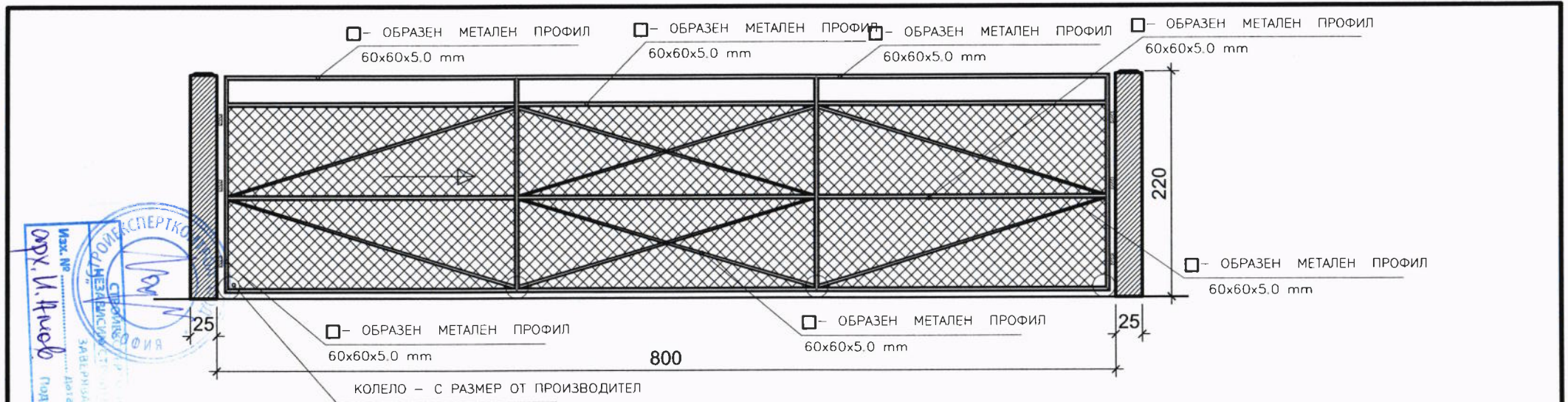
ДЕТАЙЛ НА ВХОДНА ВРАТА МАЩАБ 1: 50
