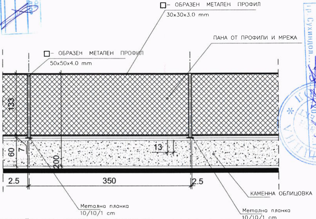
ДЕТАЙЛ НА МЕТАЛНА ОГРАДА МАЩАБ 1: 50
